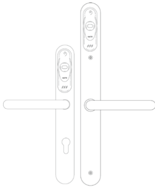
ExCD4 (beidseitig Drücker, Zylinderlochung außen)
